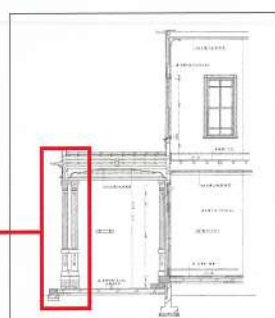
図4 研究所本館車寄せ矩計図
