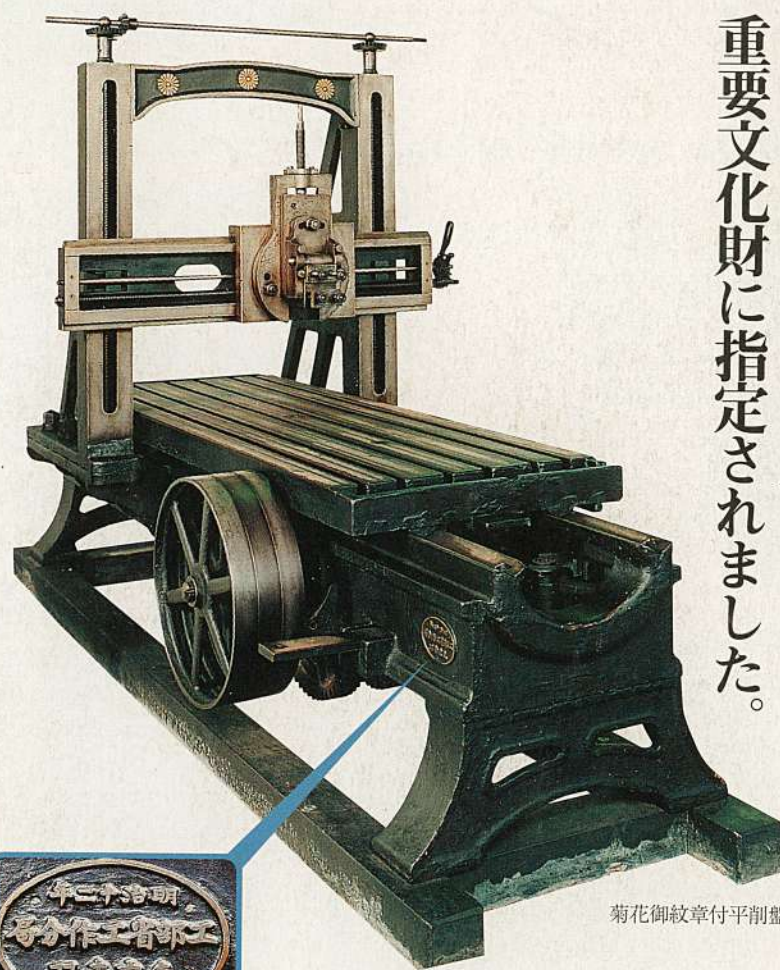
側面に取り付けられている 銘板「明治12年工部省工作 分局東京赤羽」
