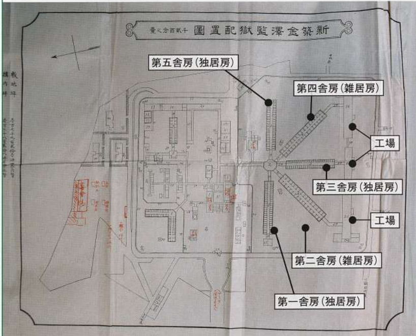
図1 新築金沢監獄配置図(「雑書編(分)冊 丙第十二類雑件」明治40年 博物館明治村保管)
