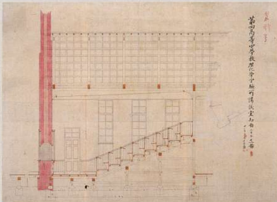
図3 第四高等学校理化学実験所講義室断面図●
