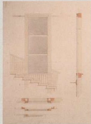
図4 理化講義室暗戸（部分）●
