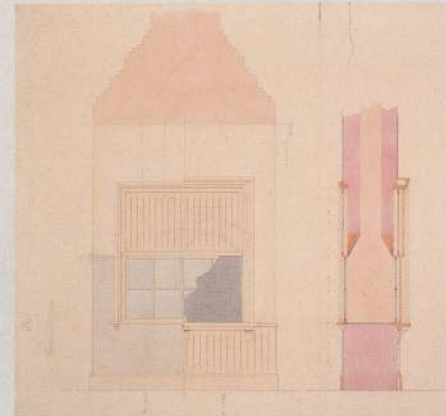
図5 理化学講義室ドラフト・チャンパー拾分之巻図（部分）●
